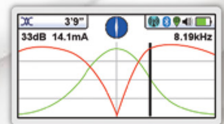
График поперечной схемы
