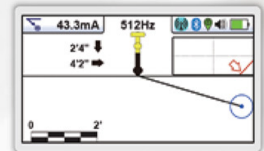
Режим бокового смещения (вектора)
