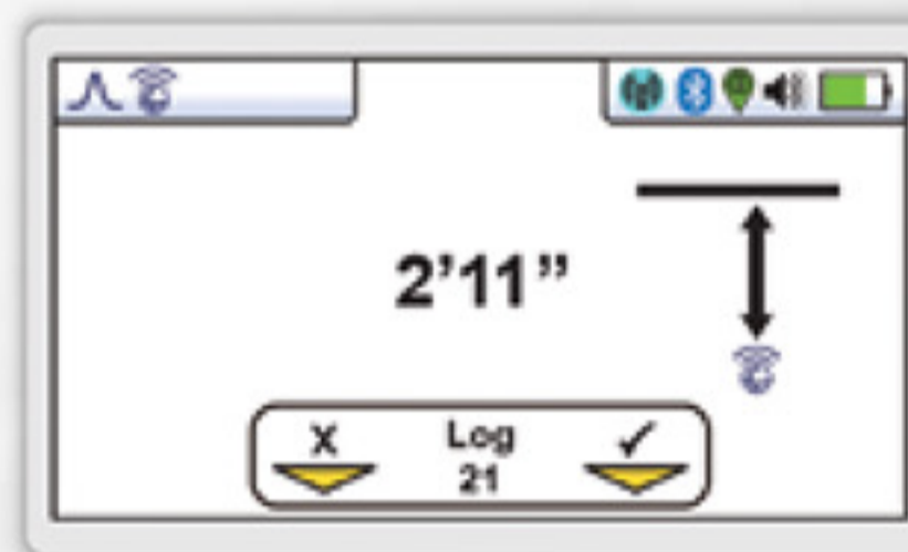
Измерение глубины маркеров и сохранение данных с GPS
